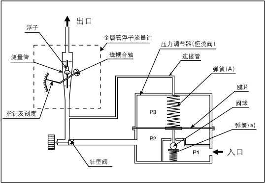
图2 测量结构示意图
