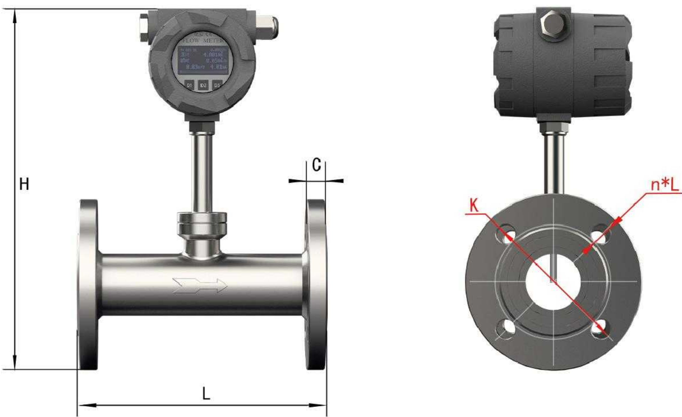
HG/T20592-2009 PN1.6Mpa(16bar)平面、突面板式平焊钢制管法兰
