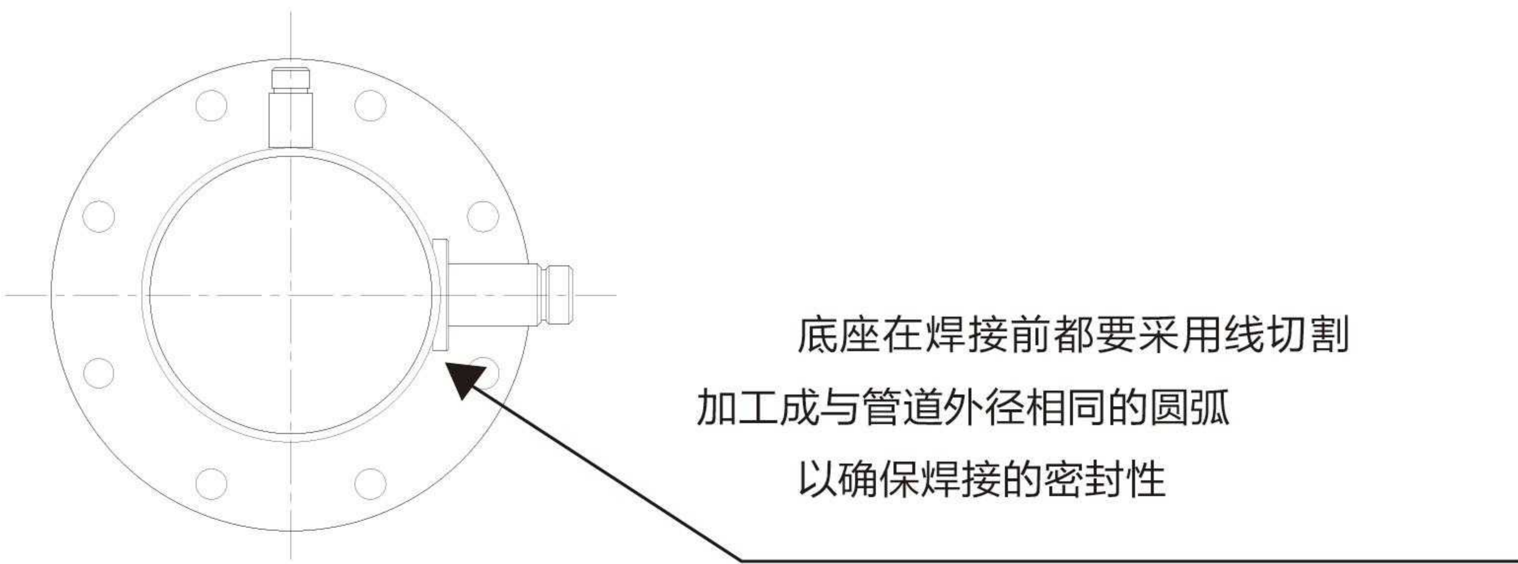
图 7 理想底座焊接位置
