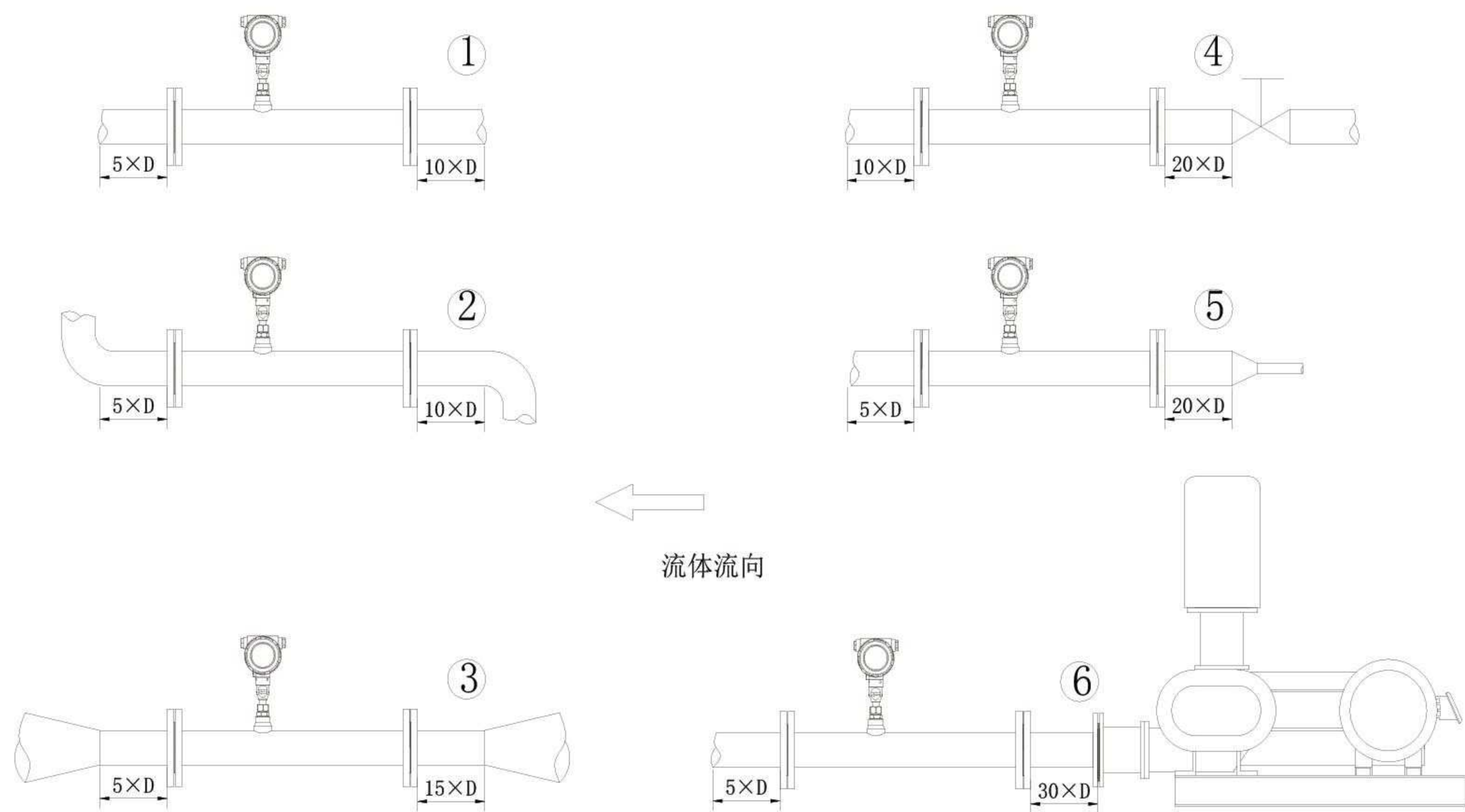
安装前后直管段图
